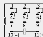
内部接线示意图
