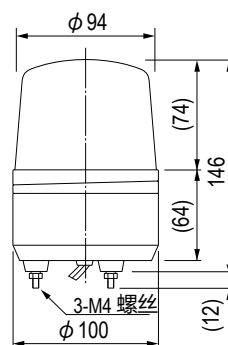
安装尺寸图
