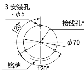
安装尺寸图
