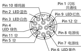
M12 接线图
