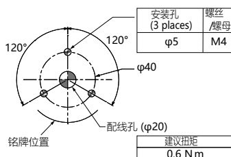
■ 【WM】安装尺寸
