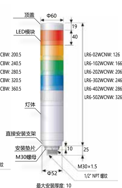
■ 【WC】安装尺寸
