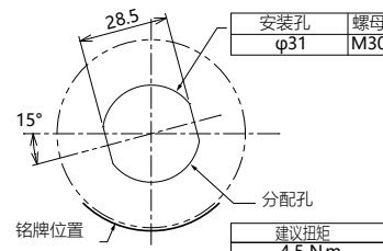
■ 【WC】安装尺寸
