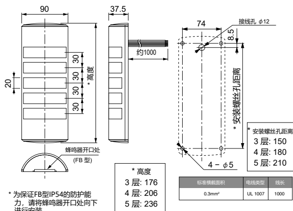
安装尺寸图
